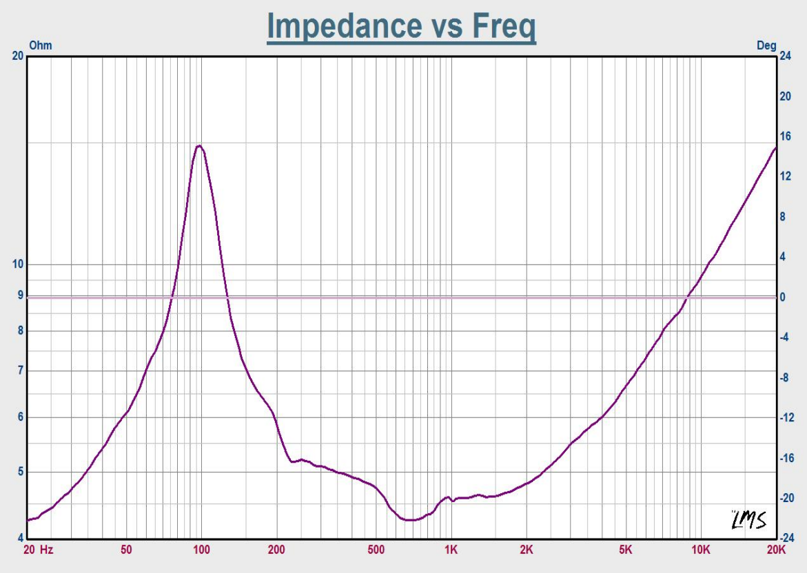
频响/阻抗曲线测试图
