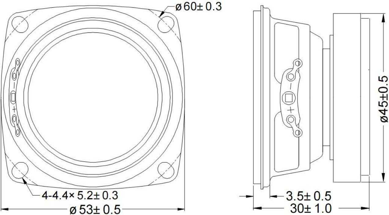
喇叭外观图
