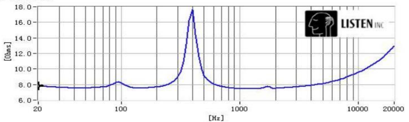
阻抗曲线
