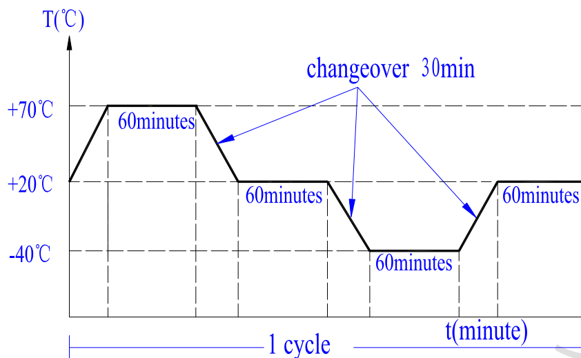
图.1. 温度循环试验
